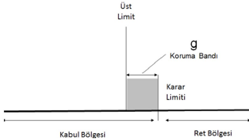
Şekil 3: Üst Limite Dayanan Kabul ve Ret Bölgesi Ölçüm sonucu karar limitine eşit ya da düşük ise uygundur.
